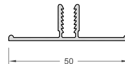
CD 112 | Basisprofiel alu CD 111 Lengte 6000 mm
