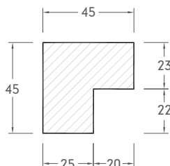
LCR 011 (3000 mm)
