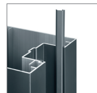
Opvulprofiel | Profil de remplissage Lengte | Longueur : 1860 mm
