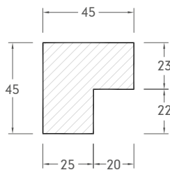
LCR 011 (3000 mm)
